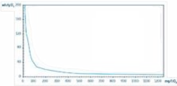
Energía eléctrica por gramo de cloro en función de la concentración de cloruros Electrical consumption per chlorine gram versus chlorides concentration Consommation électrique par gramme de chlore en fonction de la concentration en chlorures
